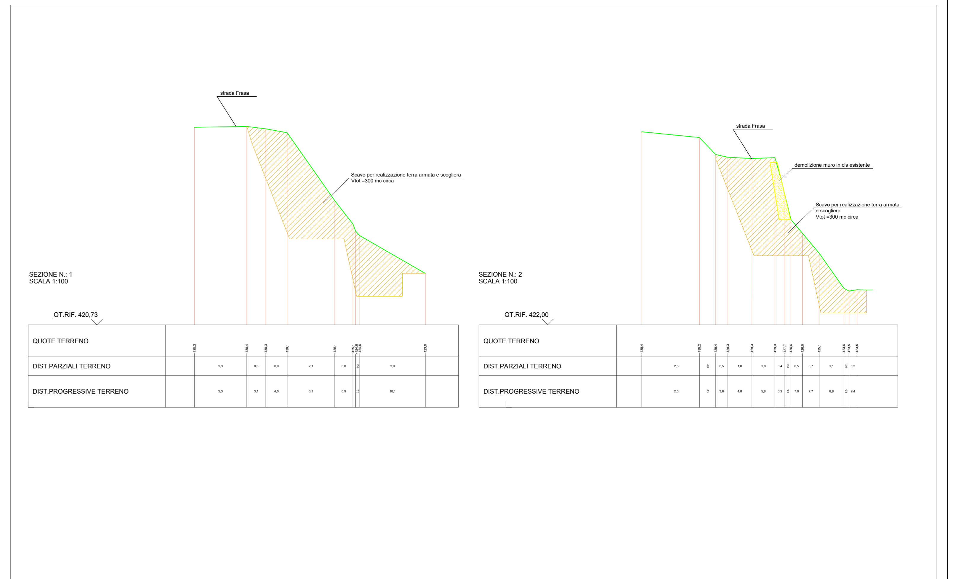
SEZIONI Stato di fatto Scala 1:100
